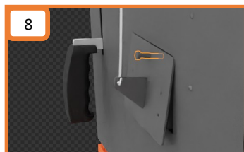
8 Minimální otevření primární klapky - klapka nesmí být nikdy úplně zavřena
