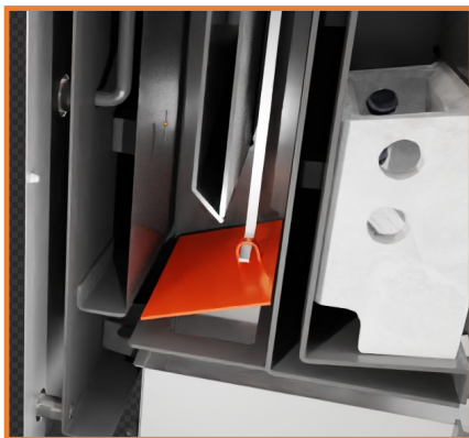
Zaháknutí čistící uzávěry pomocí čistícího nářadí (pouze NATURO 16)
